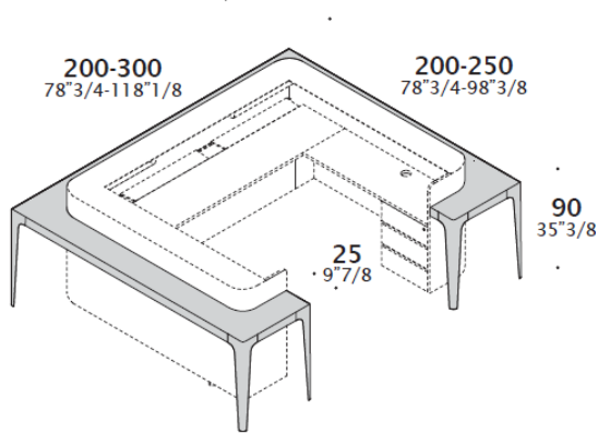
External top W200 + D200 / W300 + D250
