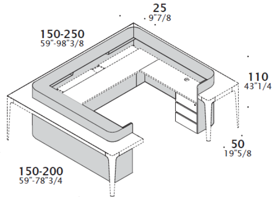
Vertical panel. W150 + D150 / W250 + D200
